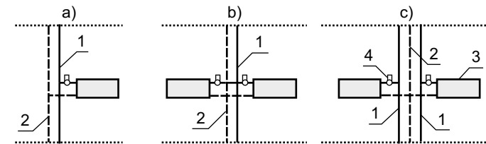
a) – iš vienos stovų pusės; b) iš abiejų stovų pusių; c) kai stovą sudaro trys vamzdžiai 1 – tiekimo stovas; 2 – grąžinimo stovas; 3 – šildymo prietaisas; 4 – termostatinis ventilis.
