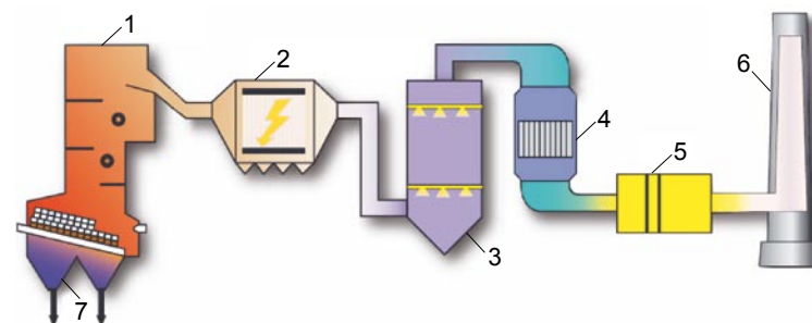
1 – katilas; 2 – elektrostatinis filtras; 3 – skruberis; 4 – azoto oksidų katalizatorius; 5 – sunkiųjų metalų ir dioksidų katalizatorius; 6 – kaminas; 7 – pelenų ir šlakų šalinimas.
